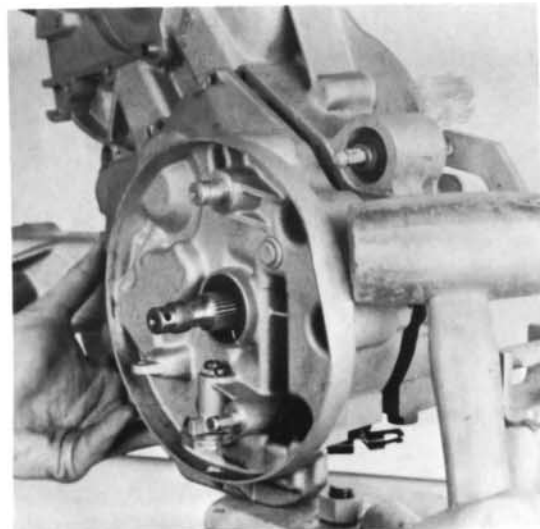
30) Gehäusehälfte abnehmen, wenn erforderlich durch leichtes Klopfen lösen.
