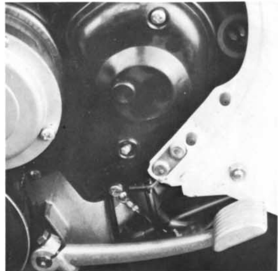
6) Schraube vom Kickstarter lösen (SW 14). Kickstarter abnehmen.
