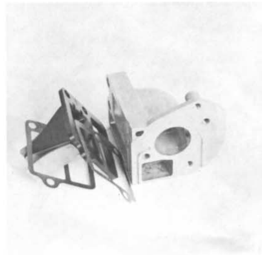
33) Membraneinlaßsteuerung mit Dichtung und Ansaugstutzen montieren. 3 Schrauben (SW 10) 6-8 Nm.
