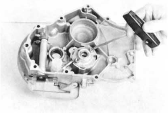
16) 2 Schrauben (SW 5) lösen.
