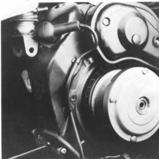
10) Befestigungsschrauben der Lüfterhaube entfernen.
