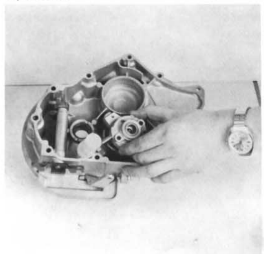
17) Hydraulikpumpe mit Filter abnehmen.
