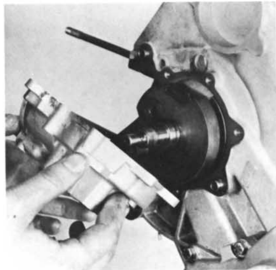
26) Gehäusehälfte, Kurbelwelle abnehmen.
