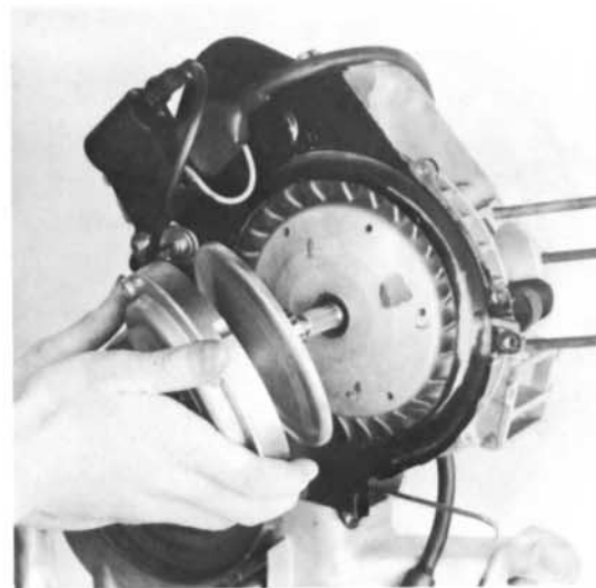
16) Kegelscheibe von der Kurbelwelle abnehmen.
