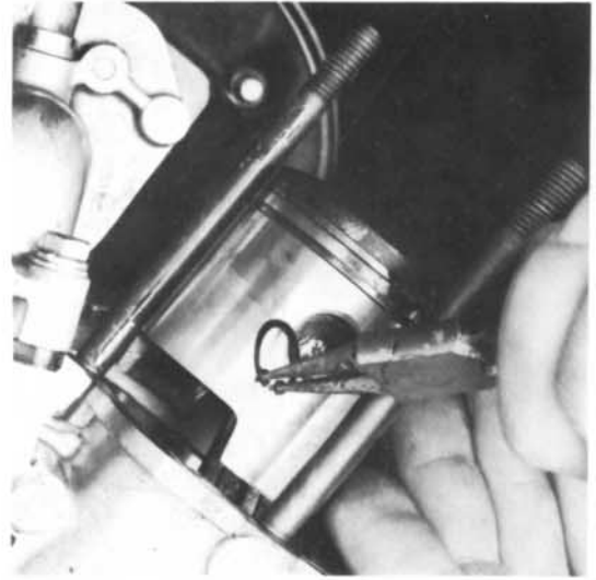
13) Kolbenbolzensicherung ausfedern.
