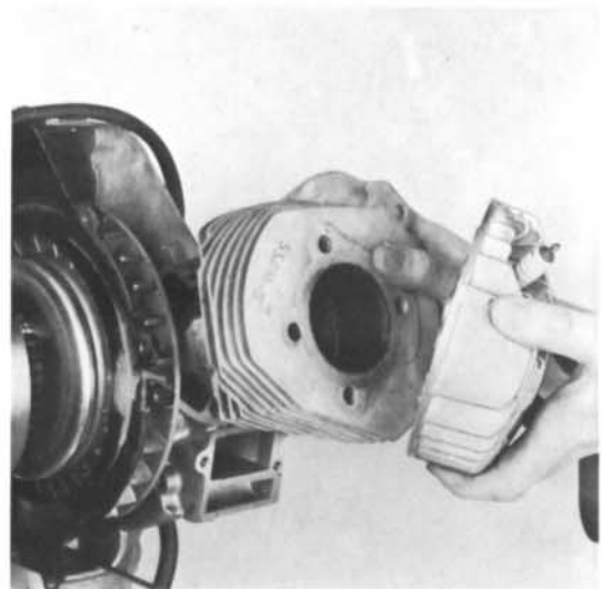
10) Zylinderkopf und Zylinder abnehmen.
