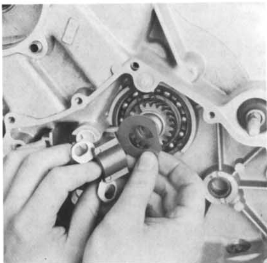
6) Scheibe und Fliehkraftregler 25-30 Nm festziehen.
