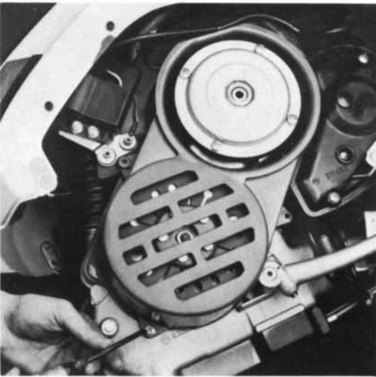
3) Gehäuseabdeckung abschrauben.
