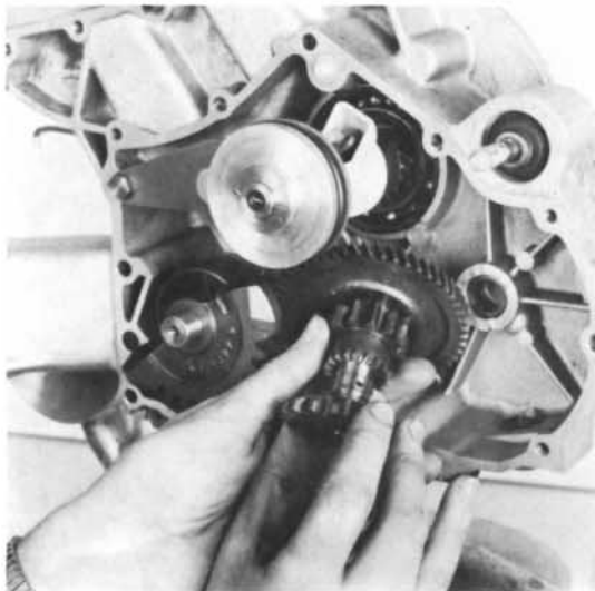
33) Vorgelegezahnrad herausziehen.
