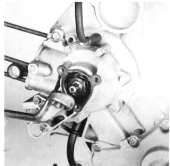
24) Mutter auf der Kurbelwelle lösen (SW 24).
