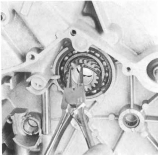
39) Sicherungsring entfernen.
