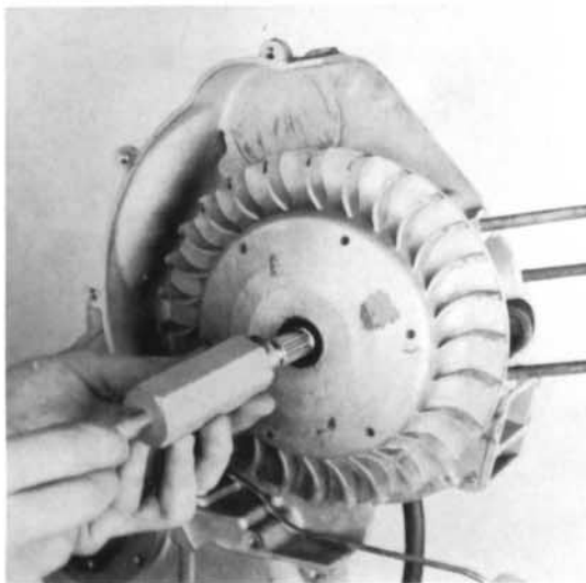
21) Polrad 19.1.20056 abziehen.
