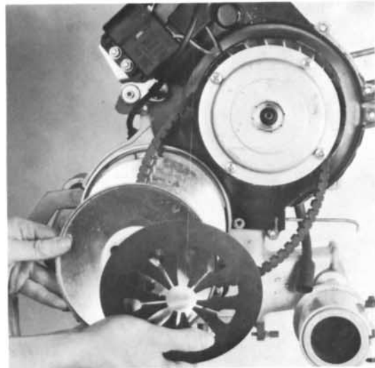
14) Tellerfeder Kegelscheibe abnehmen.
