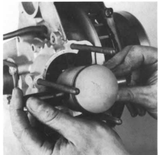
12) Kolbenbolzen herausdrücken, Werkzeugnr.: T 0017820.
