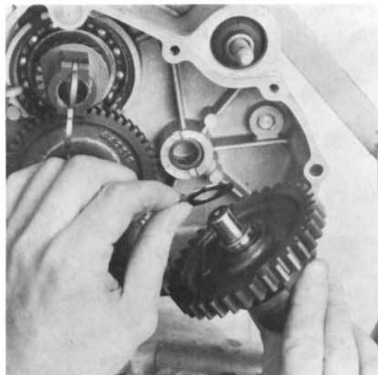
11) Scheibe montieren, Hinterachswelle einsetzen.
