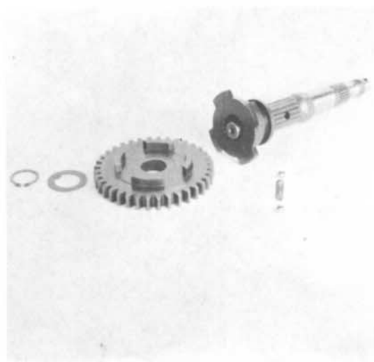
10) Seegerring und Schulterring entfernen. Zahnrad abziehen. Schiebemuffe abziehen. Mit der Hand zuhalten, damit die 2 Kugeln und die Feder nicht wegspringen können.
