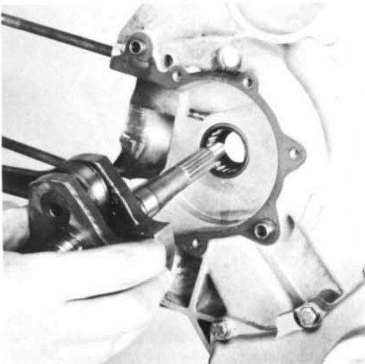
27) Kurbelwelle von Nadellager herausnehmen (3).
