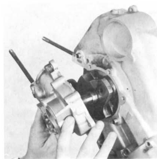
23) Gehäusehälfte mit Dichtung einsetzen. 8 Schrauben (SW 10), Federring und Scheibe einsetzen und festziehen 6-8 Nm.
