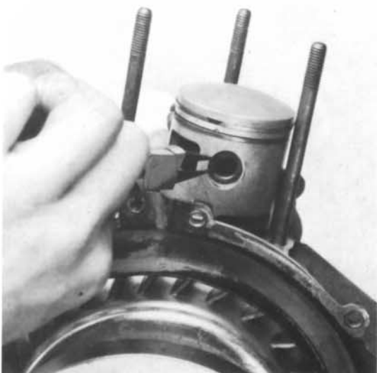
11) Beide Bolzensicherungen herausnehmen.
