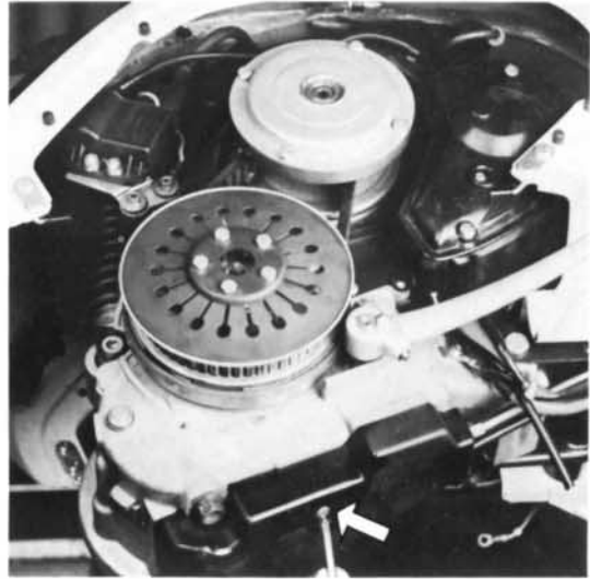
4) Abdeckkappe abschrauben.
