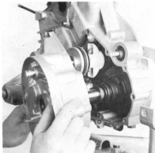
19) Gehäusehälfte aufsetzen und zusammenschrauben 6-8 Nm.
