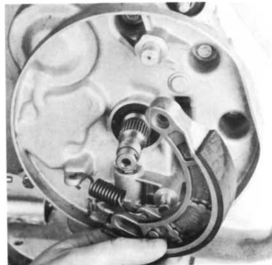
28) Beide Seegerringe abnehmen, Bremsbacken abnehmen.
