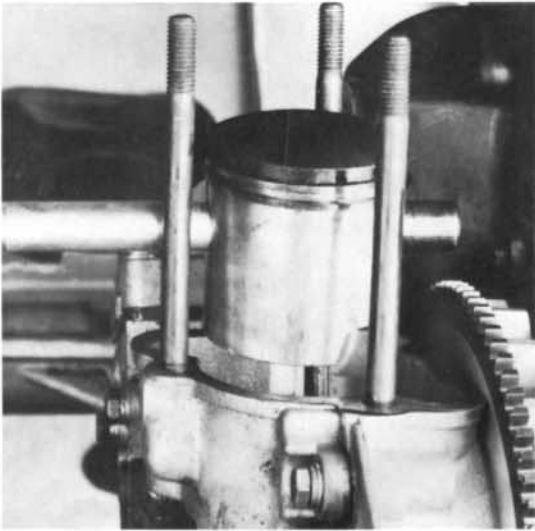
14) Kolbenbolzen mit Spezialdorn (T 0017820) herausdrücken.
