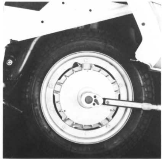
8) Kronenmutter entsplinten und abschrauben, Hinterrad mit Bremstrommel abnehmen.
