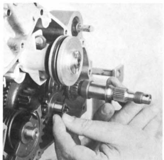
15) Anlaufscheibe einsetzen.
