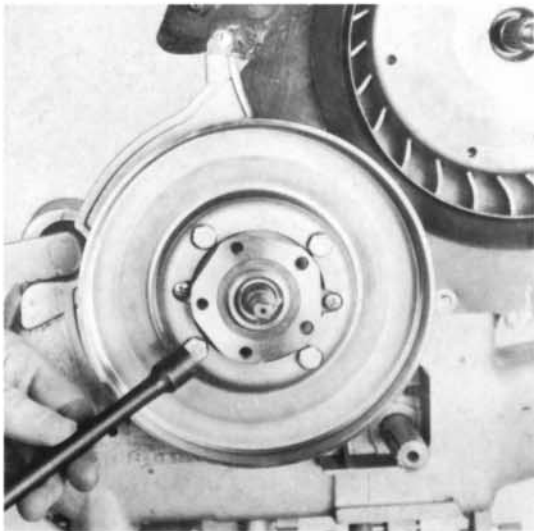
19) 4 Schrauben (SW 10) der Kupplungstrommel lösen.
