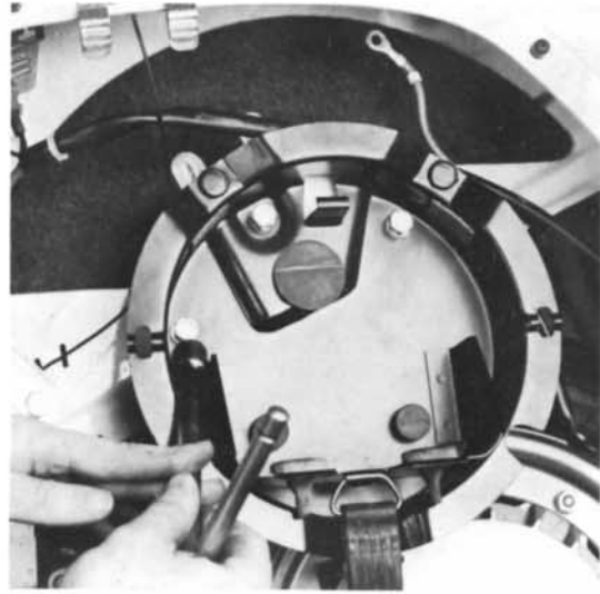
2) 4 Schrauben SW 10 lösen, Batteriehalter abnehmen.
