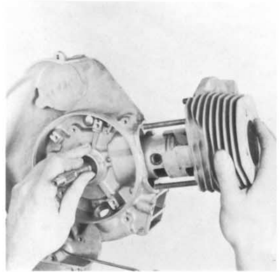
25) Fußdichtung und Zylinder montieren.
