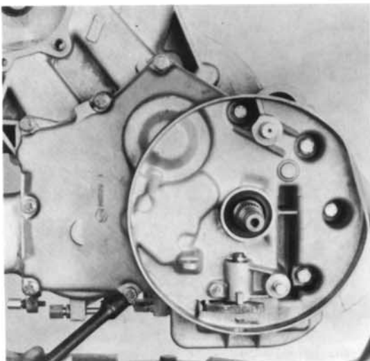
29) 11 Schrauben (SW 10) lösen.
