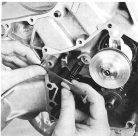
14) Gasdrehgriffbetätiger, Steuernocken und Gegen- feder einsetzen und festschrauben (SW 11 6-8 Nm) (Feder mit der engen Windung gegen das Gehäuse).
