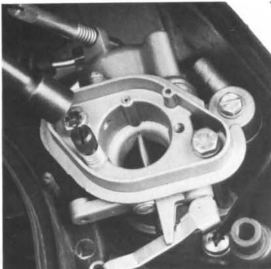
34) Vergasergehäuse (2 Schrauben) und Vergaser montieren 2 Schrauben (SW 10) 6-8 Nm.
