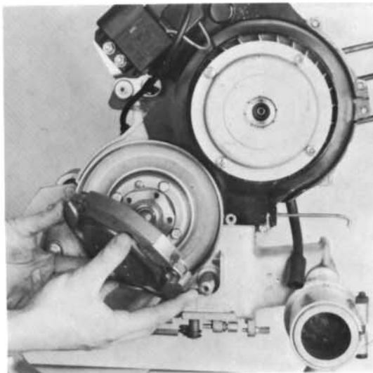
15) Kupplung abnehmen.
