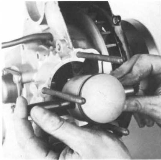
24) Kolben montieren. Pfeil nach Auslaßseite. Seegerring einfedern.
