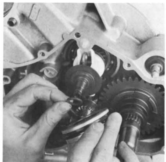
13) Distanzscheibe und Hydraulikkolben einsetzen und versplinten.
