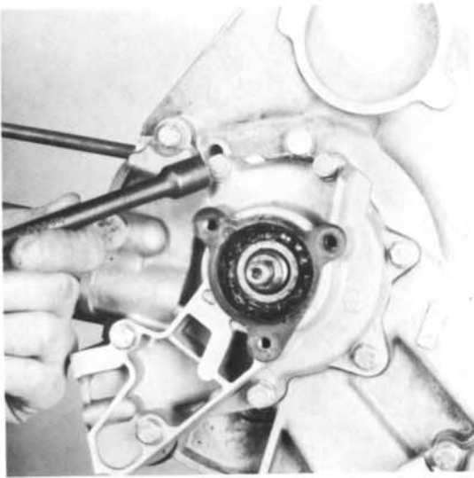
25) 7 Schrauben (SW 10) lösen.
