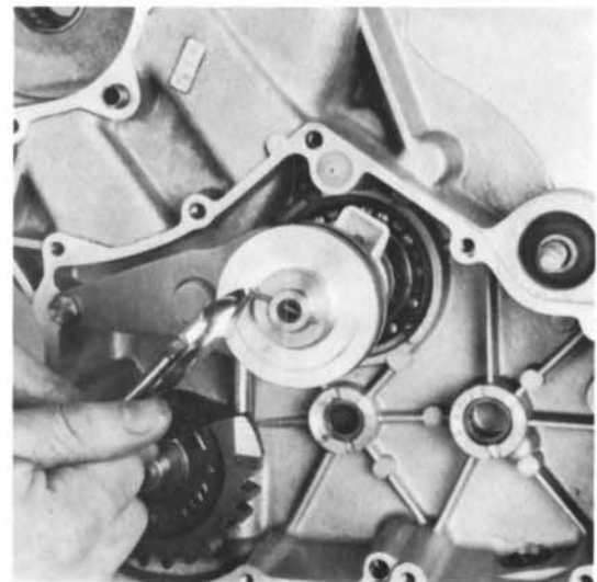
34) Steuerwelle entsplinten, Hydraulikkolben abnehmen.
