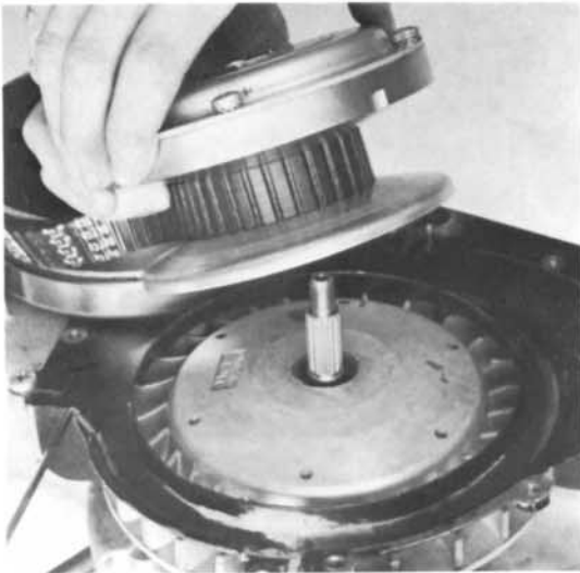
32) Zahnriemen mit Kegelscheibenhälfte einspannen und auf Kurbelwelle einsetzen. Mutter (SW 8) anziehen 40 Nm.
