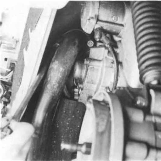
9) Schalldämpfer lösen und abnehmen.
