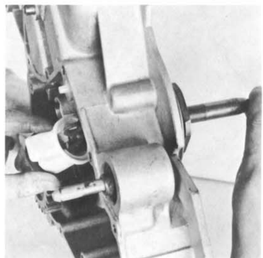
36) Steuerwelle herausziehen.
