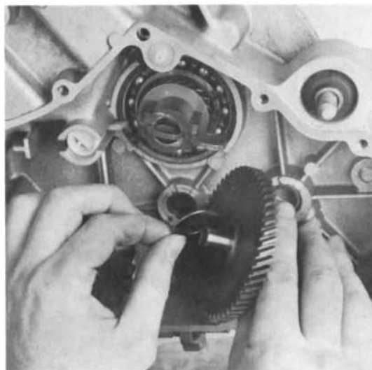
9) Anlaufscheibe auf Vorgelege montieren, Vorgelege einsetzen.
