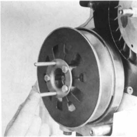
30) 5 Schrauben mit Distanzbuchse anschrauben 8-10 Nm. Mittlere Mutter von der Steuerwelle mit 35-40 Nm anziehen.
