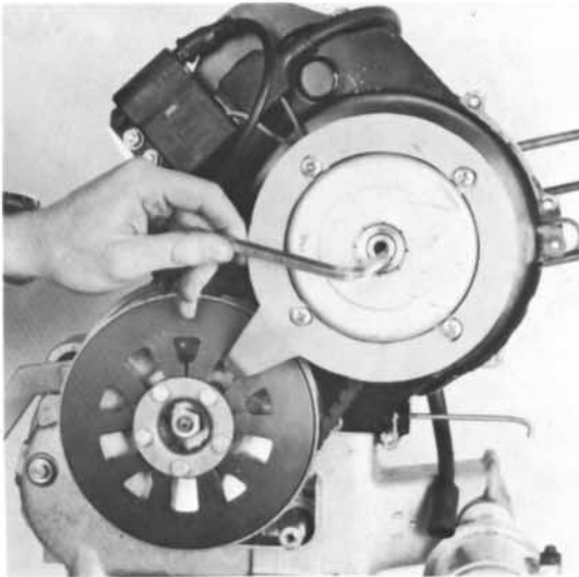
13) Werkzeug 19.1.20071 Kegelscheibenhalter, 1 Schraube (SW 8) lösen, 5 Schrauben der Tellerfeder abschrauben (SW 10), Mutter der Steuerwelle lösen (SW 17).
