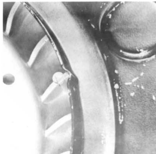
35) Zündlichtpistole anschließen. Motor starten und bei 3000 U/min. mit der Zündlichtpistole den Zündzeitpunkt kontrollieren. Der Zündzeitpunkt ist richtig, wenn die Markierung am Polrad übereinstimmt mit der Markierung am Lüfterdeckel.
