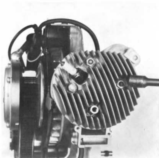
9) 4 Muttern (SW 13) von den Stiftschrauben lösen.
