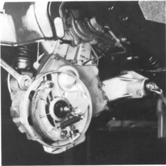
7) Traversenmutter lösen (SW 22). Untere Mutter (SW 17) für Stoßdämpferbefestigung lösen und Stoßdämpfer ausbauen.
