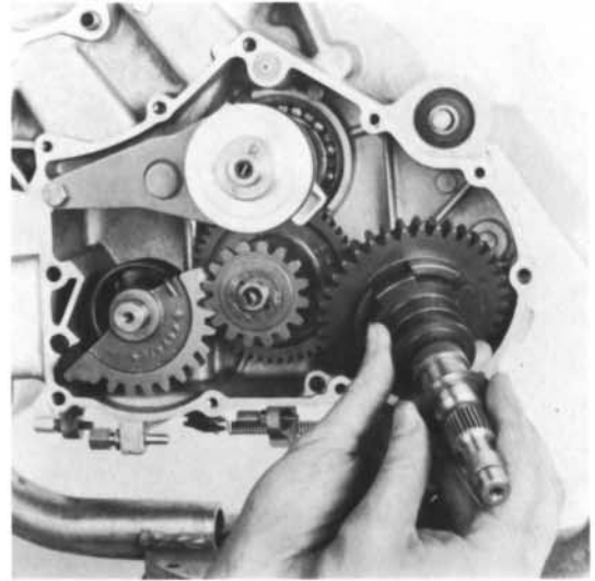
32) Hinterachswelle herausziehen.
