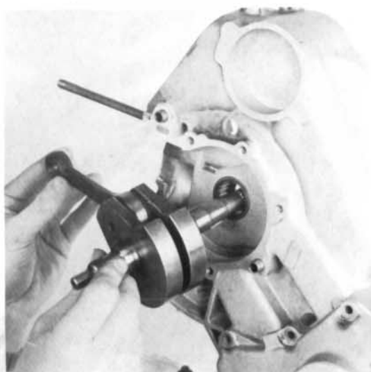
22) Kurbelwelle in Nadellager (Lichtmaschinen-seite) einführen.
