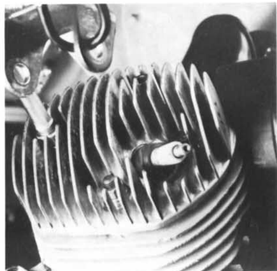
11) 3 Muttern (SW 13) und 1 Schraube (SW 13) vom Zylinderkopf entfernen.
