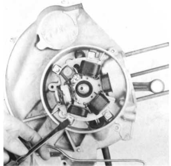
22) Lichtmaschinenankerplatte nach Lösen der 4 Befestigungsschrauben abnehmen.
