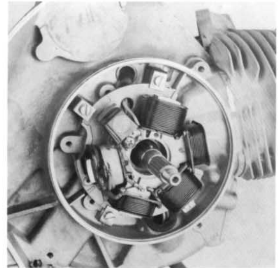
27) Ankerplatte montieren, hierbei muß die aufgegoßene Markierung für die Vorzündung am Motorgehäuse mit der Markierung an der Ankerplatte übereinstimmen. Ankerplatte festschrauben. Rotor auf Kurbelwellen- konus aufsetzen.
