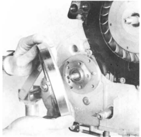
20) Kupplungstrommel abnehmen.
