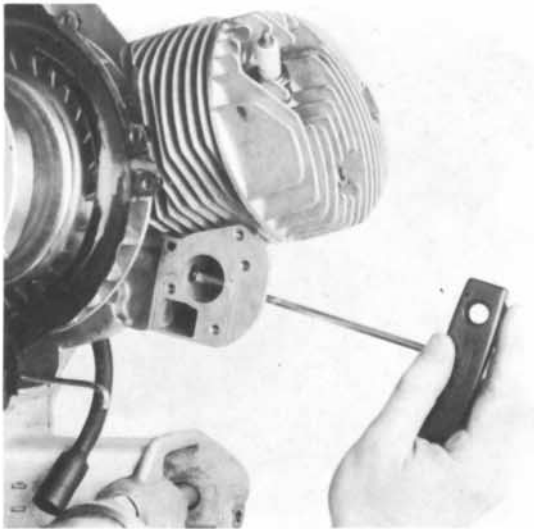
7) Mit Sechskantschlüssel (SW 5) Schraube lösen, Ansaugstutzen abnehmen.
