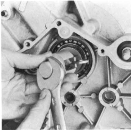
37) Fliehkraftregler mit Werkzeug 19.1.20070 abschrauben.
